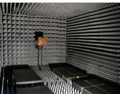
Потпуковник др Александар Ковачевић ИСПИТИВАЊЕ ЕЛЕКТРОМАГНЕТНЕ КОМПАТИБИЛНОСТИ
